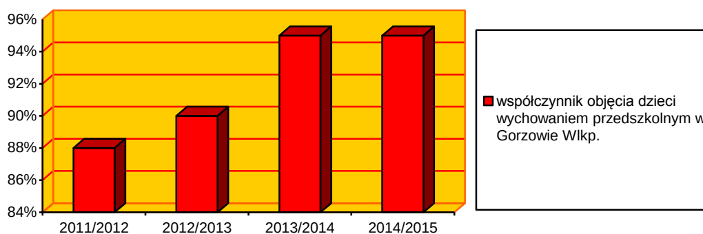
Wykres 1. Współczynnik objęcia dzieci wychowaniem przedszkolnym Gorzowie Wlkp. w latach 2011-2015.
