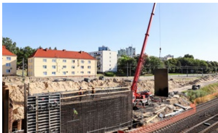
Budowa nowego wiaduktu kolejowego, Zatorze
